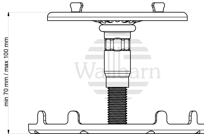
VIEW1 ( 1:2 )
