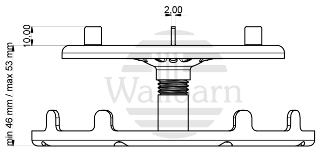
VIEW1 ( 1:2 )
