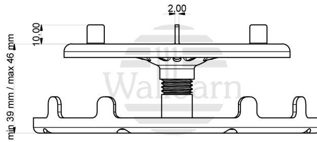
VIEW1 ( 1:2 )
