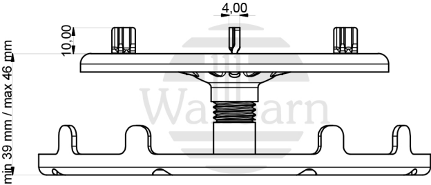
VIEW1 ( 1:2 )
