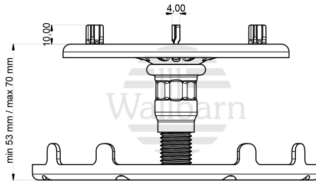
VIEW1 ( 1:2 )
