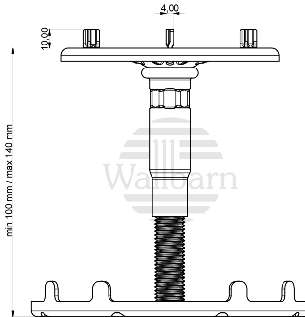
VIEW1 ( 1:2 )
